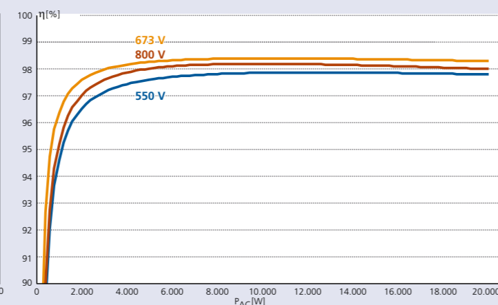
Wirkungsgradkennlinie blueplanet 20.0 TL3 INT
